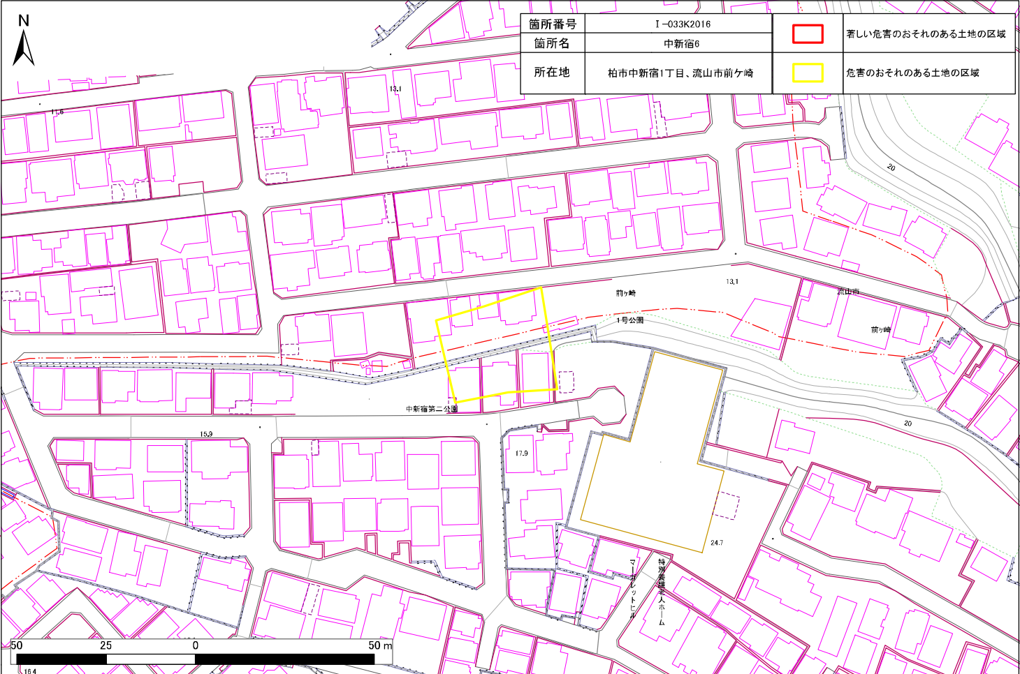
土砂災害警戒区域・特別警戒区域図(急傾斜地の崩壊) 中新宿、前ヶ崎地区
