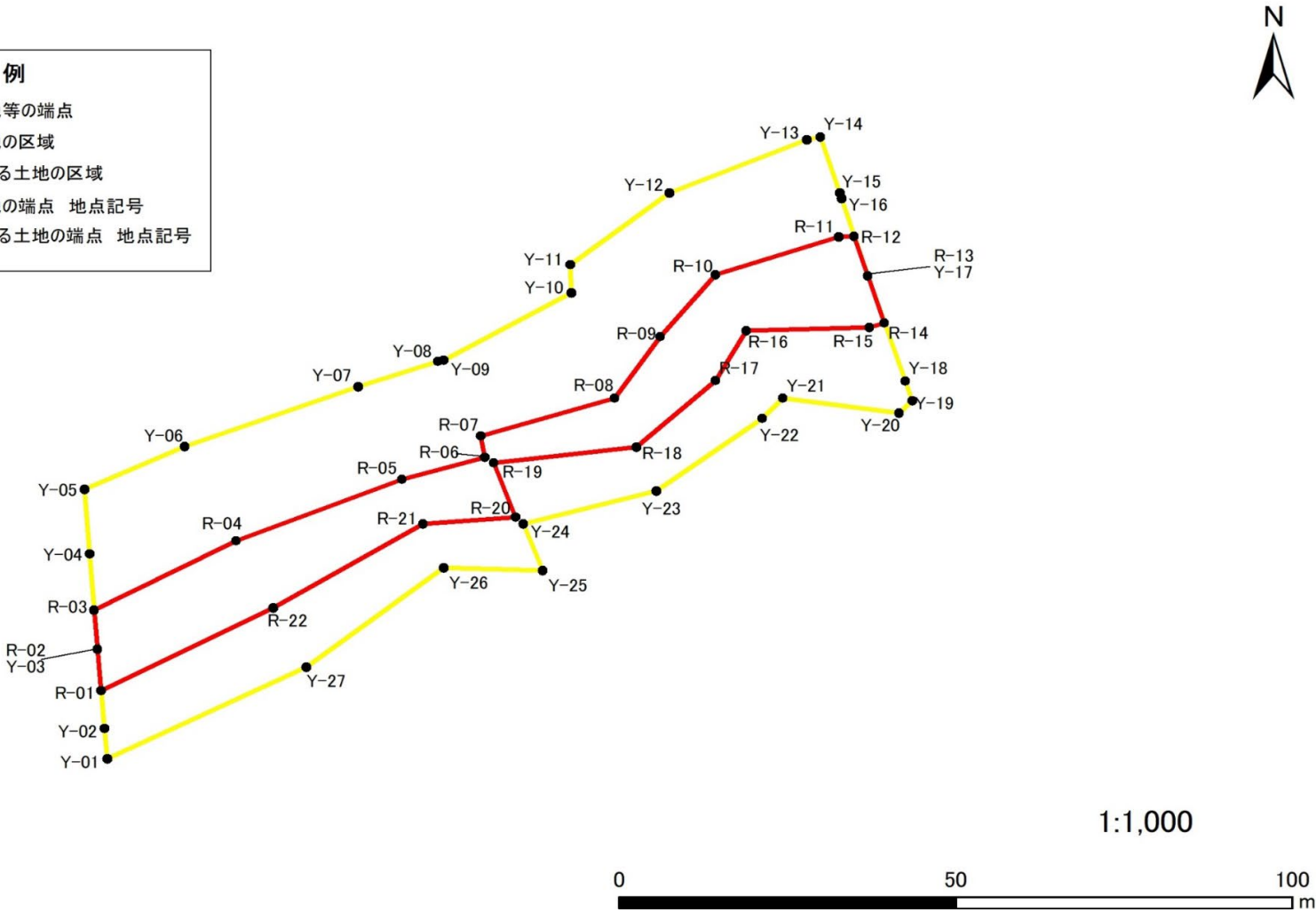
様式5-4 危害のおそれのある土地の区域の座標位置図
