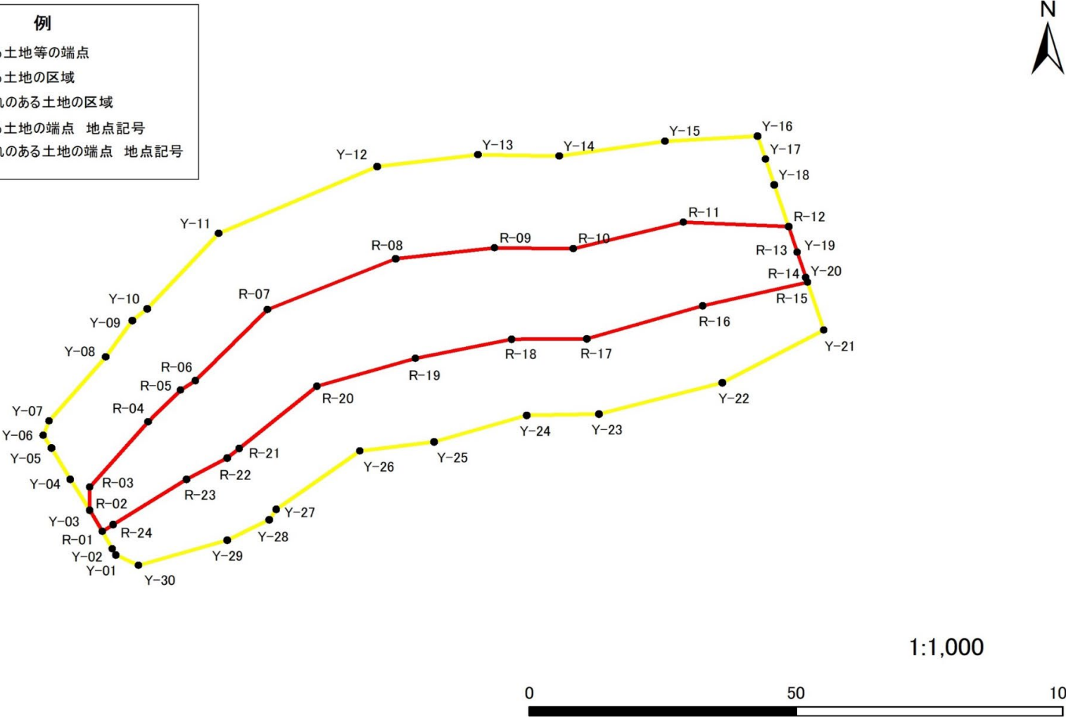
様式5-4 危害のおそれのある土地の区域の座標位置図
